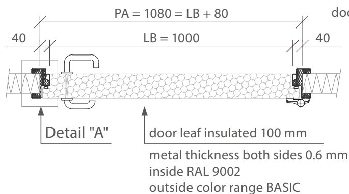
CUT A-A
